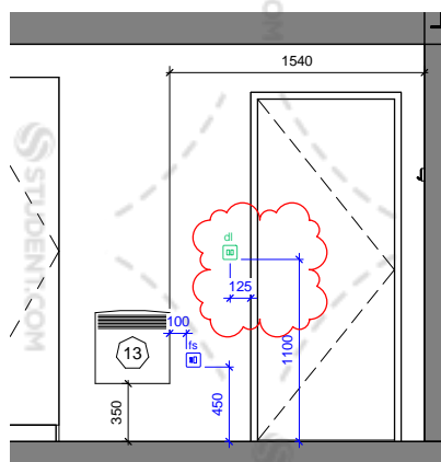
Elevation A 1 : 50
