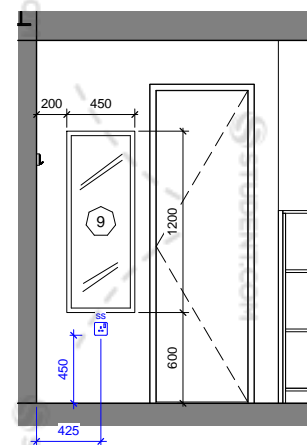
Elevation C 1 : 50
