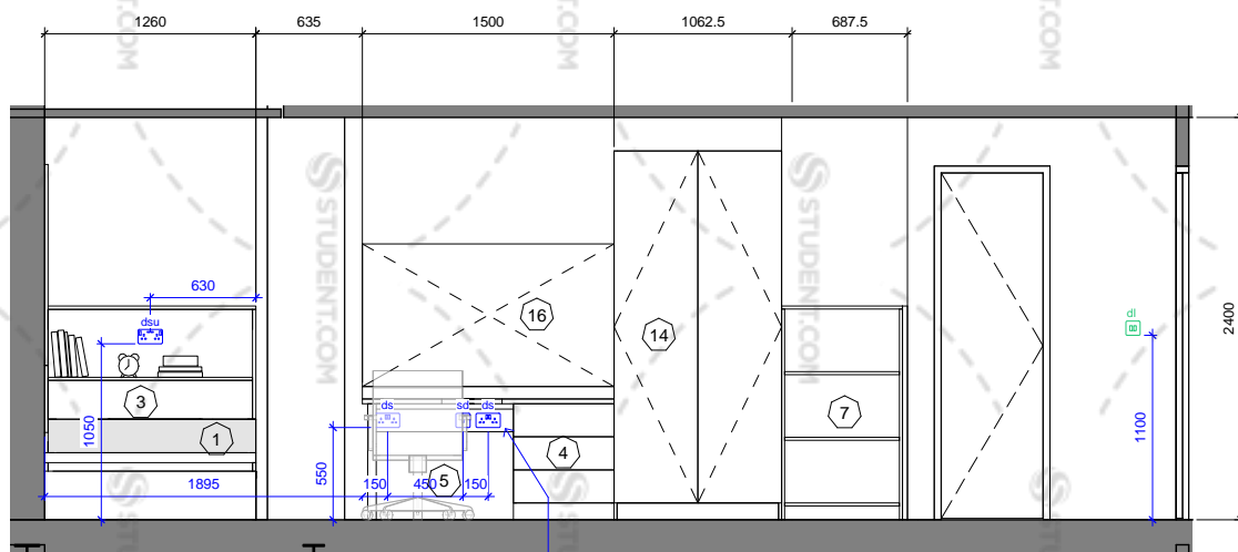
SB_4 - Elevation A
