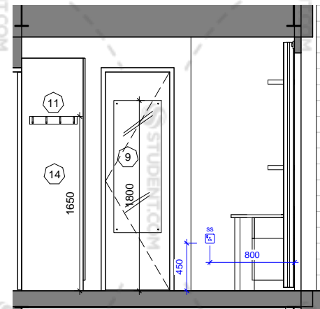
SB_11 - Elevation A
