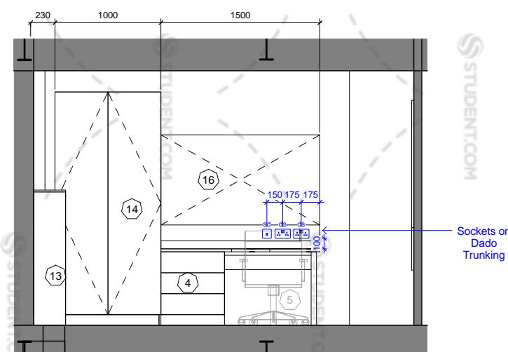
SB_12 - Elevation B
