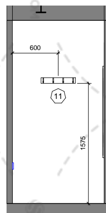
Elevations B 1 : 50
