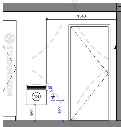
Elevation A
