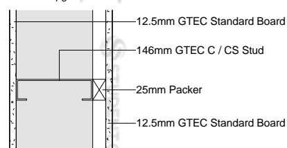
Wall Detail E 1 : 10
